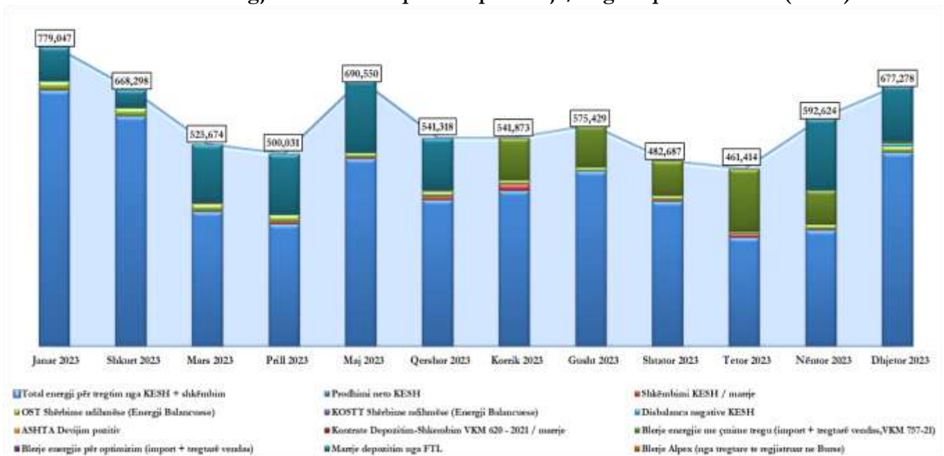
Grafiku 10. Energjia elektrike disponibël për shitje/tregtim për vitin 2023 (MWh)
