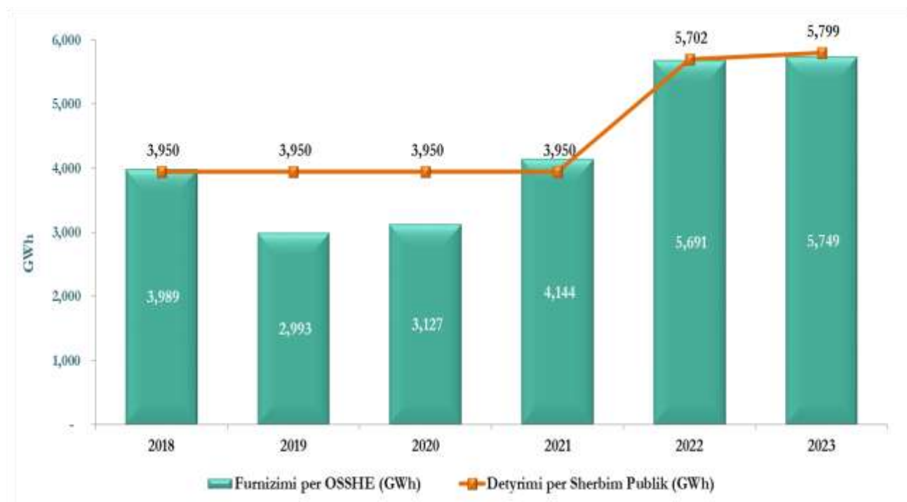
Grafiku 12. Furnizimi – Detyrimi i Shërbimit Publik 2018-2023 (GWh)
