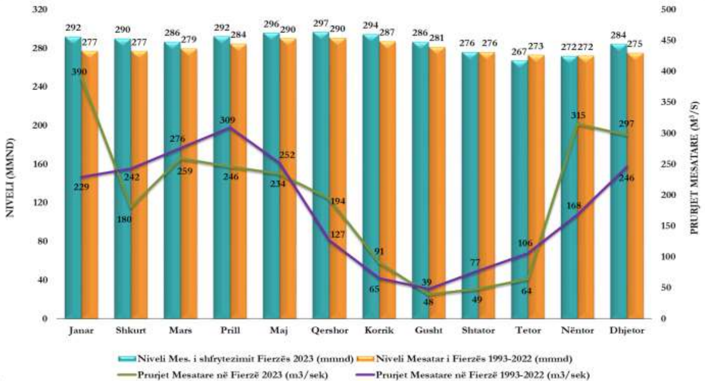
Grafiku 6. Prurjet në Fierzë dhe Niveli Mesatar i Shfrytëzimit për 2023
