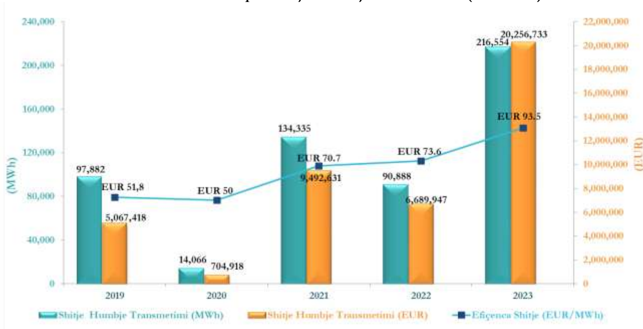
Grafiku 20. Ecuria për Shitje Humbje Transmetimi (2019-2023)
